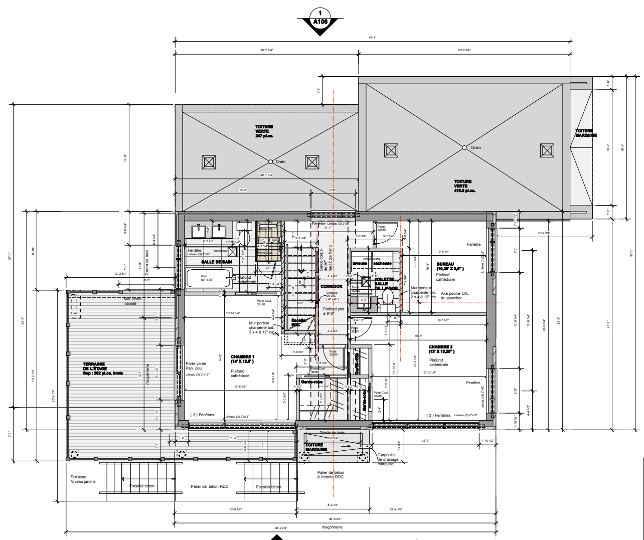
PLAN DE L'ÉTAGE Échelle : 1/4" = 1'-0"
